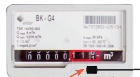
Aimant intégré dans le compteur de gaz
