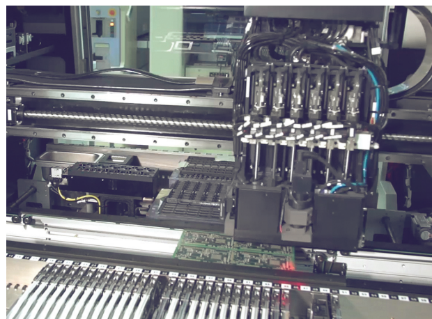
Placement de Chip
