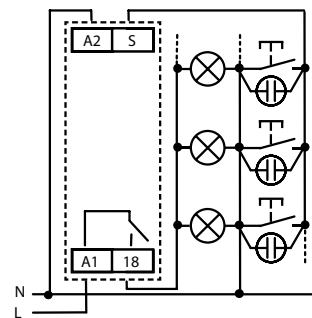
4-vodičové připojení
